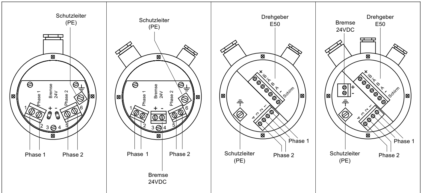
SM 56 ... Schrittmotor mit Klemmkasten
